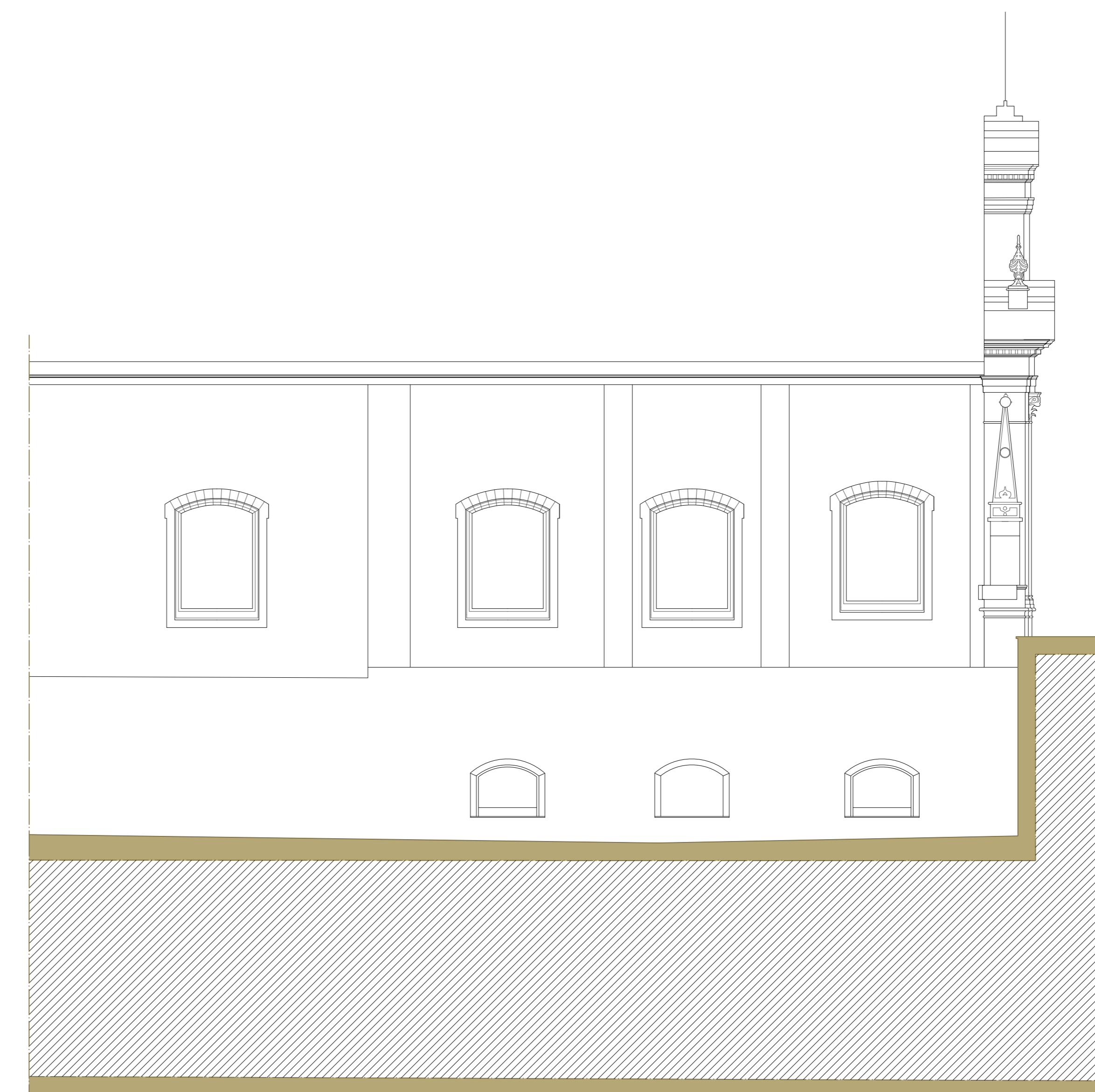
Prospetto lato Archivio
